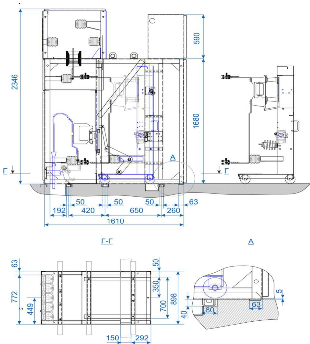
Рисунок 3 Габаритно-установочные размеры шкафа КРУ2-10
