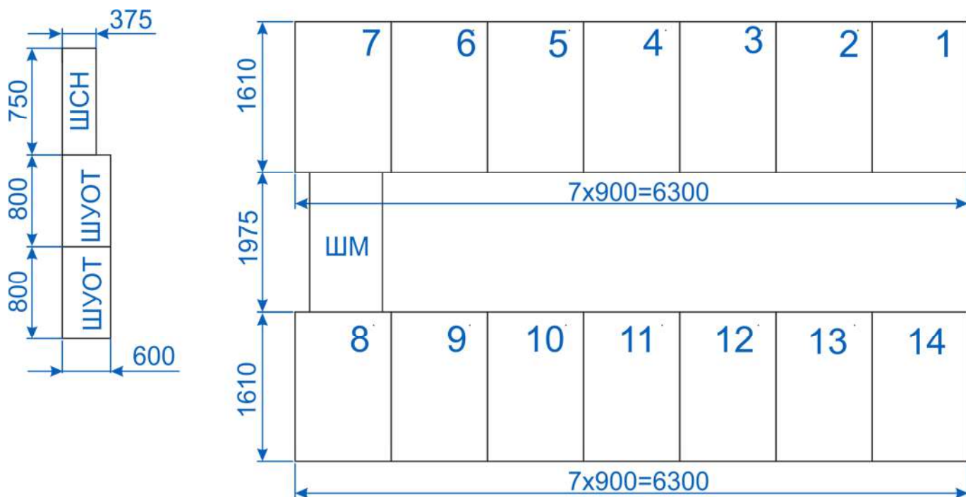
Рисунок 4 Пример плана расположения шкафов КРУ2-10 (прикладывается к опросному листу)
